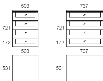
MÓDULO DE 4 CAJONES SOBRE PEANAS
