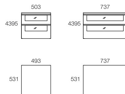
MÓDULO DE CAJÓN Y CAJÓN GRANDE COLGADO
